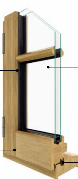
Ouvrant mouluré int. / à pente ext.
